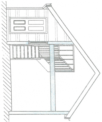
7 Section 1 1 : 50
