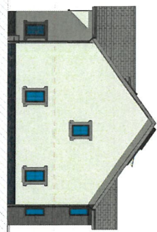
Side 1 Elevation 1:1,100
