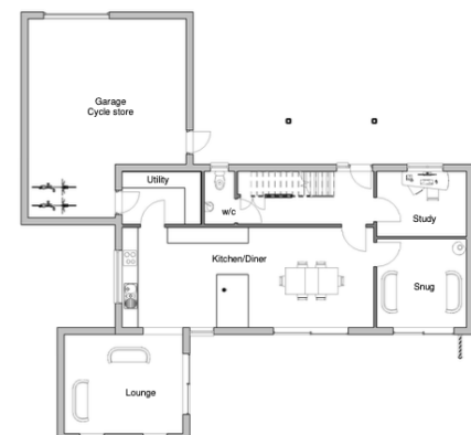
00-GF plan 1 : 100
