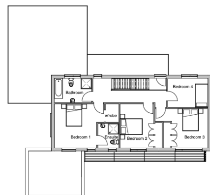
01-FF plan 1 : 100
